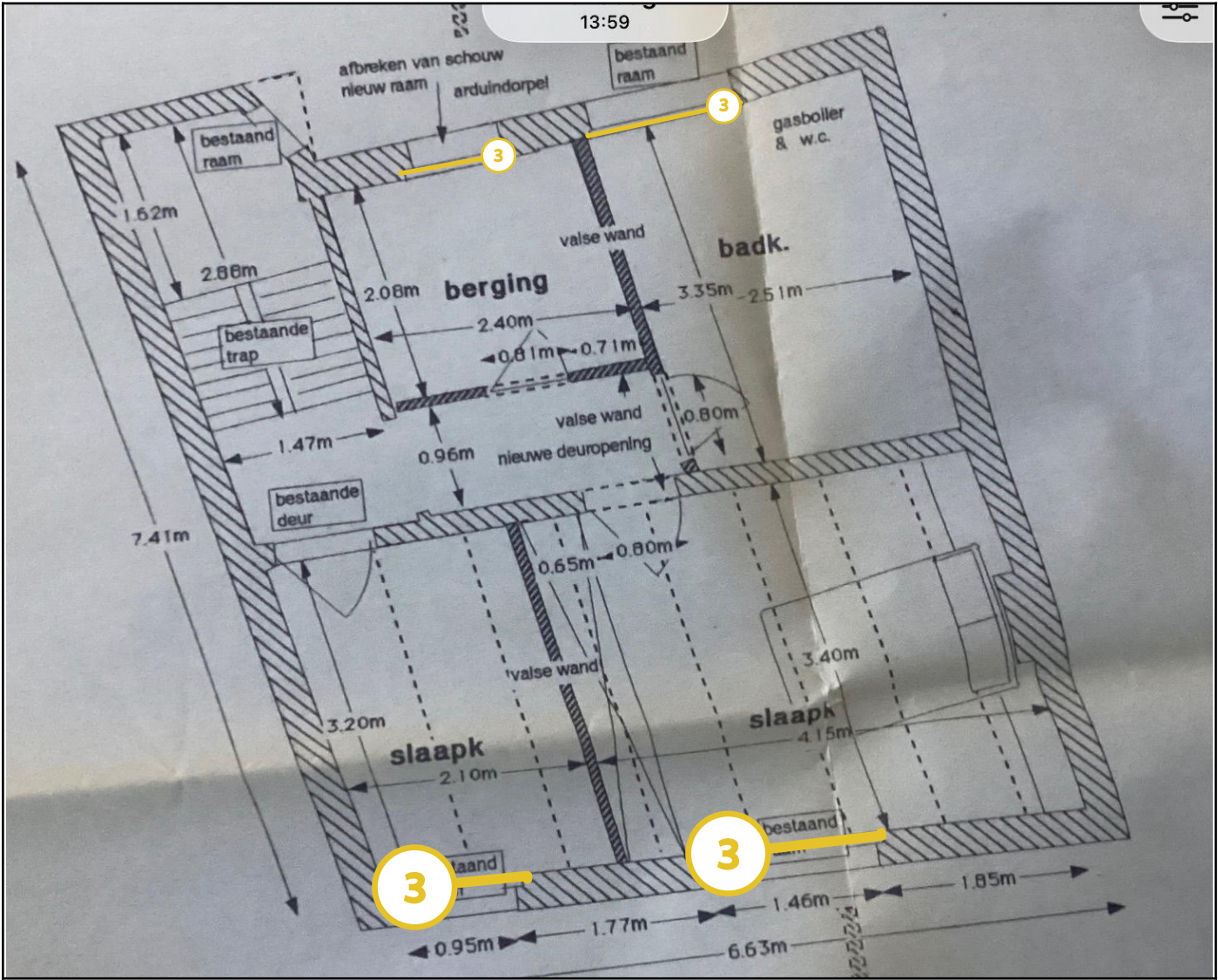
Legende van plan 1.9: Grondplan tweede verdieping
